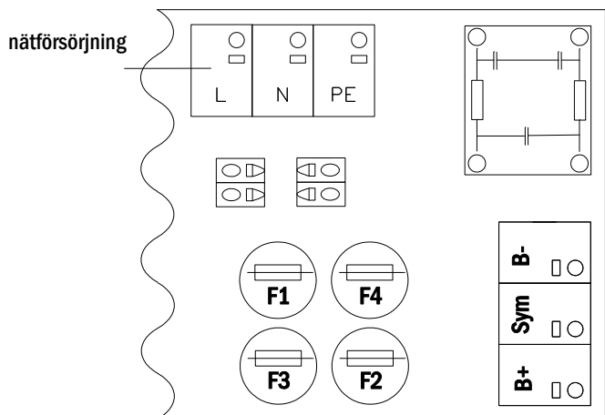
Bild 10: Nätförsörjning
