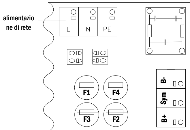
Figura 10: Alimentazione di rete
