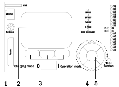
Bild 18: Styrkomponenter
