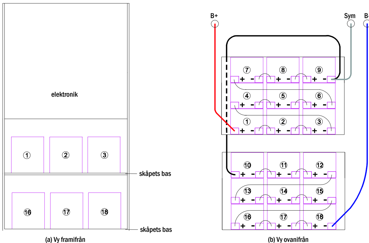
Bild 14: Montering och anslutning av batteriblock 12V 5,2Ah
