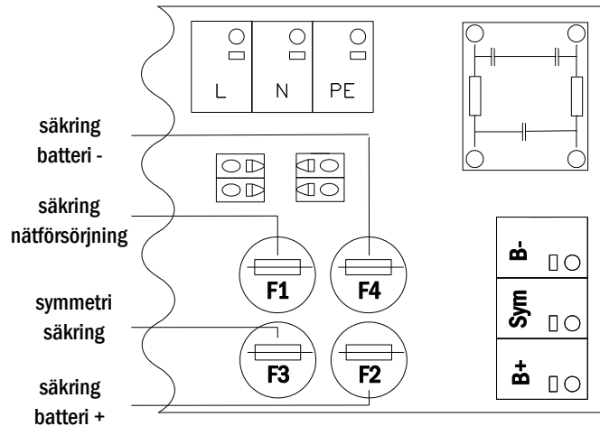
Bild 9: Säkringar nät-/batteriförsörjning
