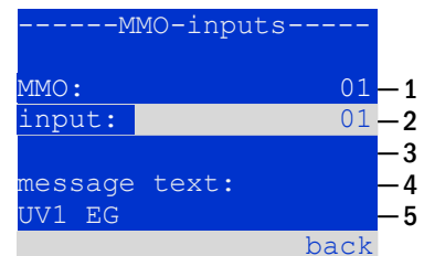
Figura 63: Programmazione ingressi MMO
