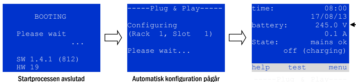
Bild 19: Startprocess (vänster, mitten) och statusmeddelande (höger).
