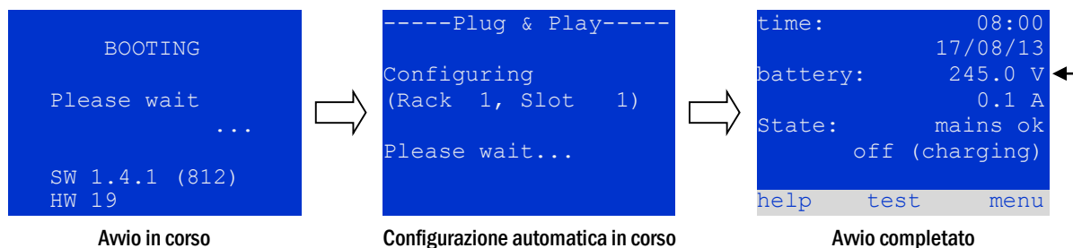
Figura 19: Processo di caricamento (sinistra, centro) e messaggio di stato (destra).
