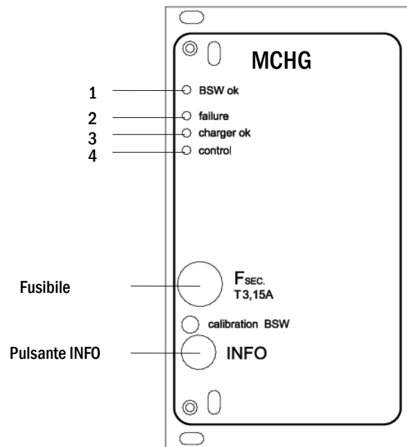
Figura 17: Modulo caricatore
