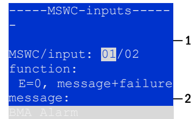
Figura 62: Programmazione ingressi MSWC
