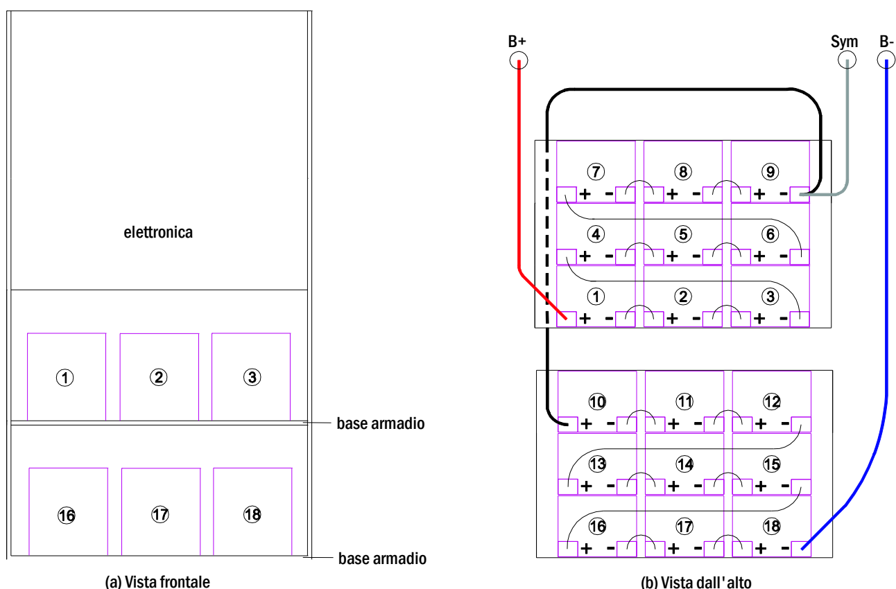
Figura 14: Montaggio e collegamento dei blocchi batteria 12V 5.2Ah
