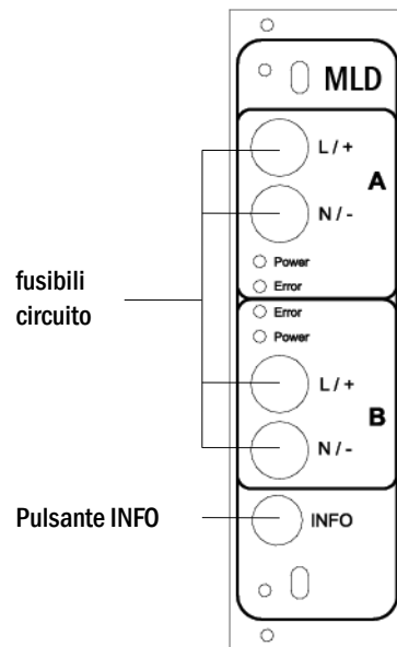
Figura 16: modulo MLD
