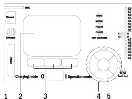
Figura 18: Elementi di comando
