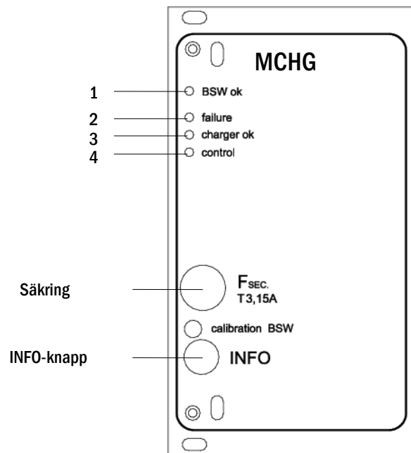
Bild 17: Laddningsmodul
