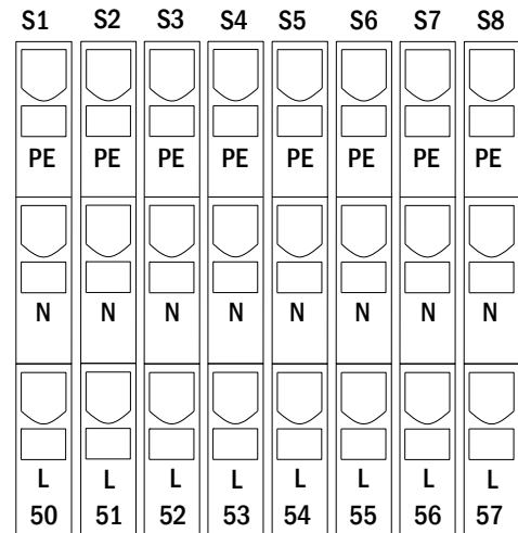
Figura 5: ingressi MMO
