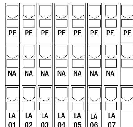
Figura 6: Linee di uscita
