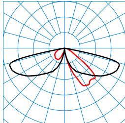
CS 19 100-AB2L-LRA/5100-740 4G1S ET (CLO end value) TX300048
