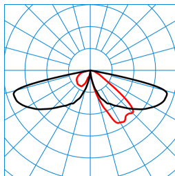
CS 19 100-AB2L-LRA/5100-740 4G1S ET (CLO initial value) TX300049
