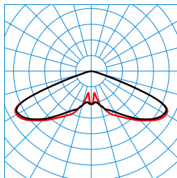
Publisca P2-RB6L-LR/4600-730 6G1S ET (CLO end value) TX301329
