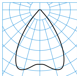
InperiaL G2 C07 BR19 2700-840 01 + ZN-PC ■ C0 - C180 TX052850
