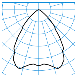
InperlaLP C05 BR22 1000-830 03 + RD-PC ■ C0 - C180 TX041534
