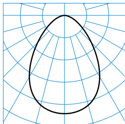
InperlaLP C05 BR22 1000-830 03 + DA-M 01 ■ C0 - C180 TX041532
