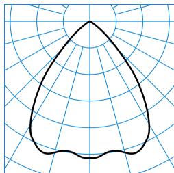
InperlaLP C05 BR22 1000-830 ET 03 ■ C0 - C180 TX771501
