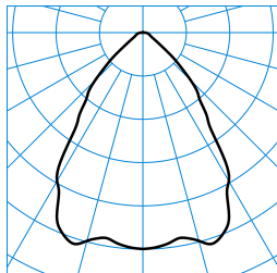
InperlaLP C05 BR22 1000-830 03 + ZN-PC ■ C0 - C180 TX041536
