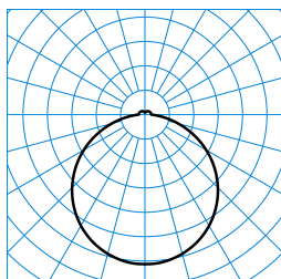
Olisq RWD4 DW 40-8TW ETBLE +CAS-S IP54 (DSU) TX876814
