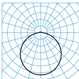
Olisq RWD4 DW 40-8TW ETBLE +CAS-S IP54 + Olisq RWD4 ZDR 1/2 01 (DWW) TX876804
