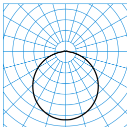
Olisq RWD4 DW 40-8TW ETBLE +CAS-S IP54 + Olisq RWD4 C 01 (DWW) TX876825
