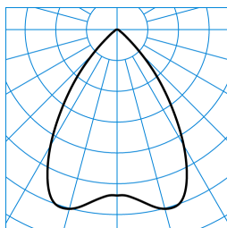
InperlaL G2 C07 HR25 4700-830 03 + RD-PC ■ C0 - C180 TX053130
