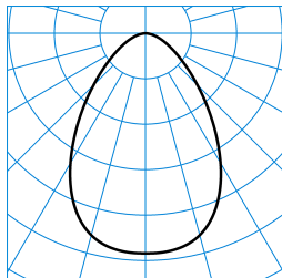
InperlaL G2 C07 HR25 4700-830 03 + DA-M 03 ■ C0 - C180 TX053129
