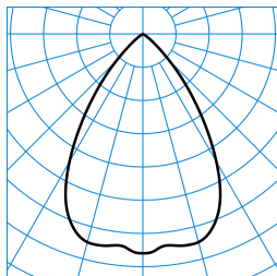
InperlaL G2 C07 HR25 4700-830 ETDD 03 ■ C0 - C180 TX770124
