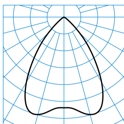
InperlaL G2 C07 HR25 4700-830 03 + DA 03 ■ C0 - C180 TX053128
