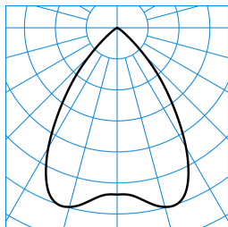
InperlaL G2 C07 HR25 3800-840 03 + DA 03 ■ C0 - C180 TX054417
