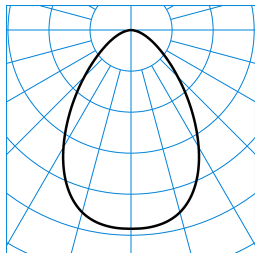
InperlaL G2 C07 HR25 3800-840 03 + DA-M 03 ■ C0 - C180 TX054418
