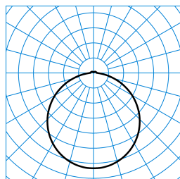
Olisq RWD4 DW 40-840 ETBLE +CAS + Olisq RWD4 ZDR 1/2 03 TX565836
