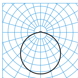
Olisq RWD4 DW 40-840 ETBLE +CAS + Olisq RWD4 ZDR 1/2 05 TX565837
