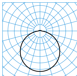
Olisq RWD4 DW 40-840 ETBLE +CAS + Olisq RWD4 ZDR 1/2 01 TX565835
