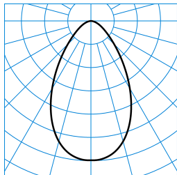
InperlaLP C05 HR22 2700-830 01 + DA-M 01 ■ C0 - C180 TX041714
