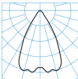
InperlaLP C05 HR22 2700-830 01 + RD-PC ■ C0 - C180 TX041716
