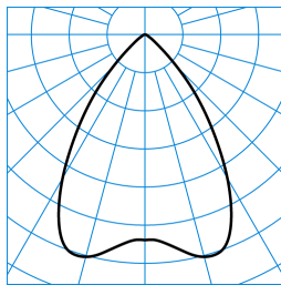
InperlaL G2 C07 HR19 1000-830 01 + RG-PC ■ C0 - C180 TX052981
