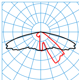
Publisca P1W-AB2L-LR/1800-730 2G1S ET (CLO end value) TX301945
