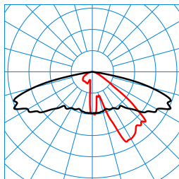
Publisca P1W-AB2L-LR/1800-730 2G1S ET (CLO initial value) TX301277
