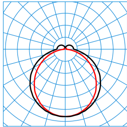
Olisq LWD3 DW 50-830 ETDD IP54 PC TX376051
