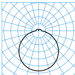
Olisq RWD2 DW 40-8TW ETDD8 IP54 PC (DSU) TX873689
