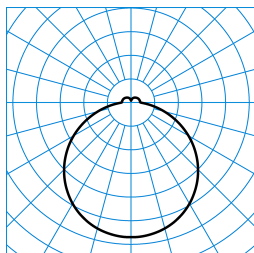
Olisq RWD2 DW 40-8TW ETDD8 IP54 PC (DWW) TX873690
