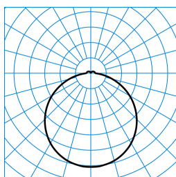
Olisq RWD2 DW 40-8TW ETDD8 IP54 PC + RWD2 ZDR 1/2 01 (DWW) TX873700
