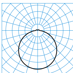
Olisq RWD2 DW 40-8TW ETDD8 IP54 PC + RWD2 ZDR 1/2 03 (DWW) TX873703
