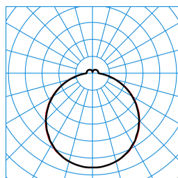
Olisq QWD2 DW 14-40/4/ML-830 IP54 ET (stage 1) TX777789
