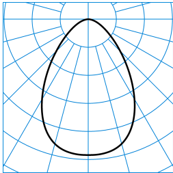
InperlaL G2 C07 HR19 1800-830 01 + DA-M 01 ■ C0 - C180 TX053003
