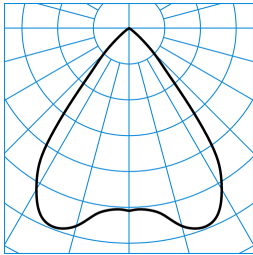
InperlaL G2 C07 HR19 1800-830 ETDD 01 ■ C0 - C180 TX769465
