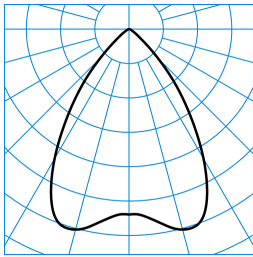
InperlaL G2 C07 HR19 1800-830 01 + RG-PC ■ C0 - C180 TX053005
