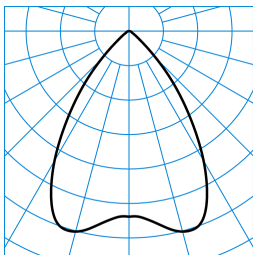
InperlaL G2 C07 HR19 1800-830 01 + RD-PC ■ C0 - C180 TX053004
