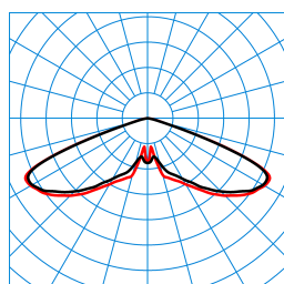
Publisca P2-RB6L-LRA/3200-730 4G1S ET (CLO initial value) TX301590
