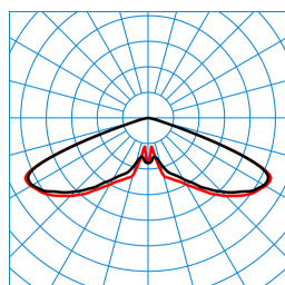
Publisca P2-RB6L-LRA/3200-730 4G1S ET (CLO end value) TX301873
