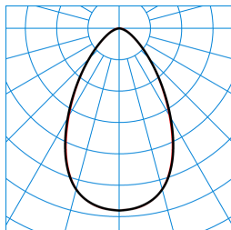
7651IP MironaF TB 270-840ET L225 01 (LEO1) TX306194
