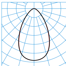
7651IP MironaF TB 270-840ET L225 01 (LEO3) TX306196
