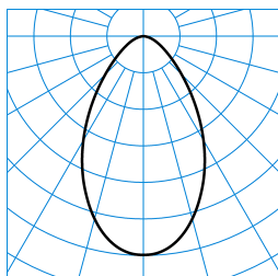
InperlaLP C05 BR19 1800-830 03 + DA-M 01 ■ C0 - C180 TX041513
