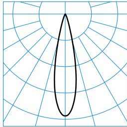
7651 Lentyp L-SP 40-835 M34 ETBLE 01 (150) TX782526
