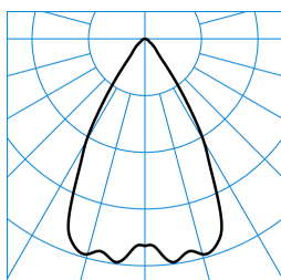
InperlaLP C05 HR22 2700-830 03 + RG-PC ■ C0 - C180 TX041724
