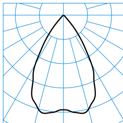
InperlaLP C05 HR22 2700-830 ETDD 03 ■ C0 - C180 TX771307
