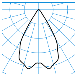
InperlaLP C05 HR22 2700-830 03 + ZN-PC ■ C0 - C180 TX041725
