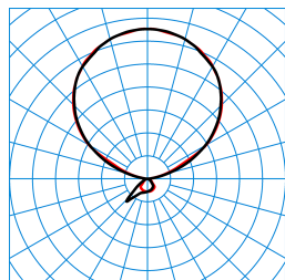
Luceos S-U PAW-IL 170-840 ETDD 05 (LEO2) TX877125
