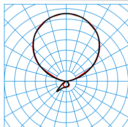
Luceos S-U PAW-IL 170-840 ETDD 05 (LEO1) TX877133
