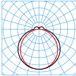
Olisq LWD3 DW 30-830 ET HFS IP54 TX430088
