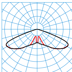
Publisca P2-RB6L-LR/1200-740 2G1S ET (CLO initial value) TX301130
