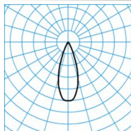
SNS RC3-HR1FL-14-940
