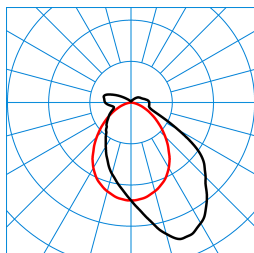
TugraHE 15 PAW 60-8TW ETDD8 01 (DWW) TX876987
