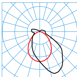
TugraHE 15 PAW 60-8TW ETDD8 01 (DSU) TX876991
