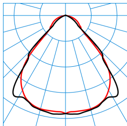
SFlow C2-L MRW LED4000-840 ET 01 TX771498
