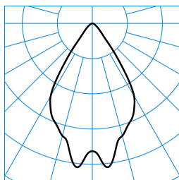
InperlaLP C05 BR19 1800-840 03 + RD-PC ■ C0 - C180 TX041233
