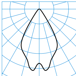
InperlaLP C05 BR19 1800-840 03 + ZN-PC ■ C0 - C180 TX041235
