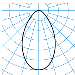
InperlaLP C05 BR19 1800-840 03 + DA-M 03 ■ C0 - C180 TX041232
