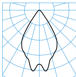
InperlaLP C05 BR19 1800-840 03 + RG-PC ■ C0 - C180 TX041234
