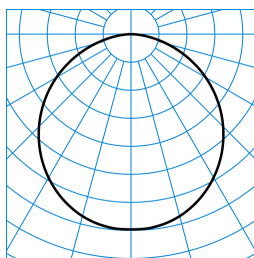
Olisq RWD3 DW 30-840 ETBLE +DMR IP54 + Olisq RWD3 ZDR 1/1 01 TX426585
