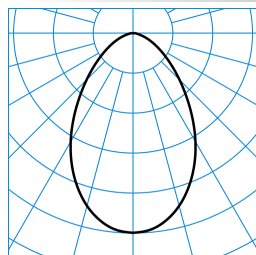
Ambiella G2 C07 WR LED2000-840 ET 01 TX773103 ■ C0 - C180
