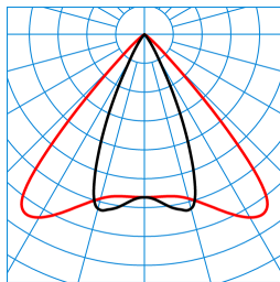
E-Line 7651 Grado WRS-DF84 50-EC M47 ETDD 03 (225) TX845404
