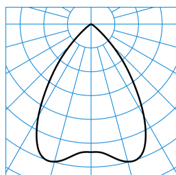
InperlaL G2 C07 BR19 2700-830 01 + DA 01 ■ C0 - C180 TX052834
