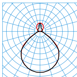
Luceos D/H1-L CDP 4000-8TW ETDD 03 (Ceiling D1 ZD/03) (DWW) TX877230
