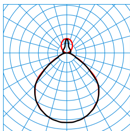
Luceos D/H1-L CDP 4000-8TW ETDD 03 (Ceiling D1 ZD/03) (DSU) TX877229
