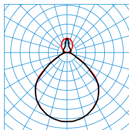
Luceos D/H1-L CDP 4000-8TW ETDD 03 (Ceiling D1 ZD/03) (DCW) TX877228
