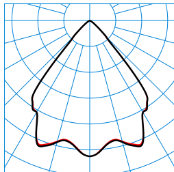
Creavo M73-TS LW19-03 30-840 ETDD 01 TX781771
