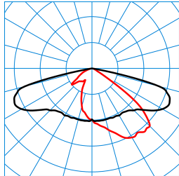
LIQ 70N-AB7L-LR/16000-730 12G1 ET (CLO end value) TX778252
