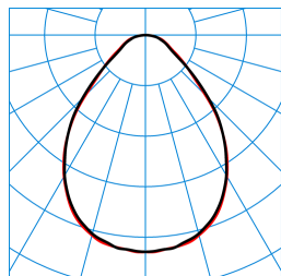
ArimoFit G2 M57 PW19 42-830 ETDD + ArimoFit G2 Sky M57-TS ZER TX426369
