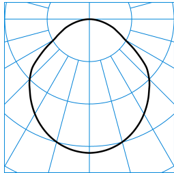
Inplana C07 OTA25 2000-840 01 + C07 ZPF - T ■ C0 - C180 TX772427
