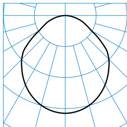
Inplana C07 OTA25 2000-840 01 + C07 ZPF - T WR ■ C0 - C180 TX772429
