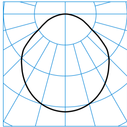
Inplana C07 OTA25 2000-840 ETDD 01 ■ C0 - C180 TX772431
