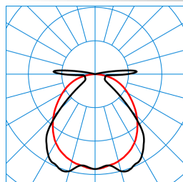
OleveonF 12 B 4000-840 ETDD +DMM TX770085
