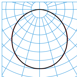
Olisq QWD3 DW 30-840 ET EB3 IP54 IK + Olisq QWD3 ZDR 1/1 01 TX460743
