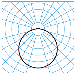
Olisq QWD2 DW 35-840 ETBLE +DMM IK + Olisq QWD2 ZDR 1/2 01 TX461952
