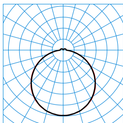
Olisq QWD2 DW 35-840 ETBLE +DMM IK + Olisq QWD2 ZDR 1/2 03 TX460744
