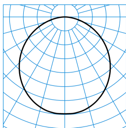
Olisq RWD1 DW 10-840 ETBLE +CAS IP54 + Olisq RWD1 ZDR 1/1 01 TX565911
