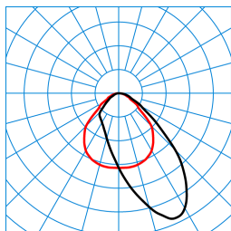
Luceos D/H2-L CDP-A 5000-840 ETDD 01 (Pendant ZS/ZST+EB3) TX877154
