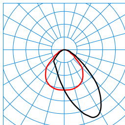
Luceos D/H2-L CDP-A 5000-840 ETDD 01 (Ceiling D2 ZD/01+EB3) TX877152
