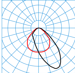
Luceos D/H2-L CDP-A 5000-840 ETDD 01 (Ceiling D2 ZD/01) TX877270
