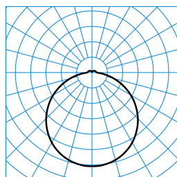
Olisq RWD2 DW 40-8TW ETDD8 IP54 + RWD2 ZDR 1/2 05 (DWW) TX873687
