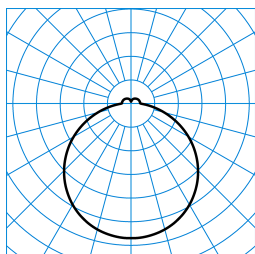
Olisq RWD2 DW 40-8TW ETDD8 IP54 (DSU) TX873665
