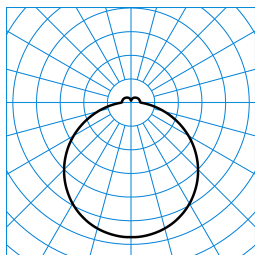
Olisq RWD2 DW 40-8TW ETDD8 IP54 (DWW) TX873666
