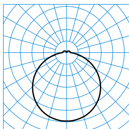
Olisq RWD3 DW 30-840 ETBLE +DMM PC + Olisq RWD3 ZDR 1/2 05 TX426230
