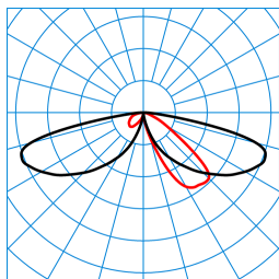
LTX LT-AB2L-LRA/15/18/26-730 4G1 (1800 lm) TX084095
