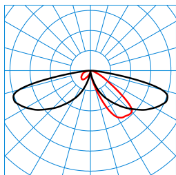
LTX LT-AB2L-LRA/15/18/26-730 4G1 (2600 lm) TX084096
