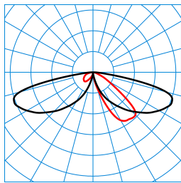
LTX LT-AB2L-LRA/15/18/26-730 4G1 (1500 lm) TX084094
