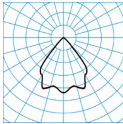
ELINE HE CLW2240-120 ML 840 L225 2 20 ■ C0 - C180 DIN 5040 = A60 UGR I 3 = 20,3 UGR q 3 = 20,4 UTE 3 = 1.00 A CEN flux code = 89 100 100 100 100
