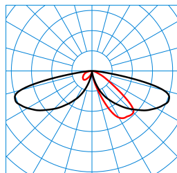
LTX KT-AB2L-LR/3800-730 4G1 ET TX780676
