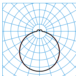
Olisq QWD2 DW 14-40/4/ML-830 ET IK (stage 3) TX842839
