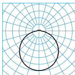
Olisq QWD2 DW 14-40/4/ML-830 ET IK + Olisq QWD2 ZDR 1/2 01 (stage 0) TX842885
