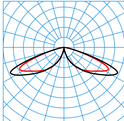
LTX ZT-RB6L-LRA/1800-740 2G1 ETDD TX779398
