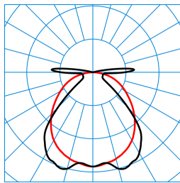
AragF 12 PW 44-840 ET PC RCY +LV TX830177
